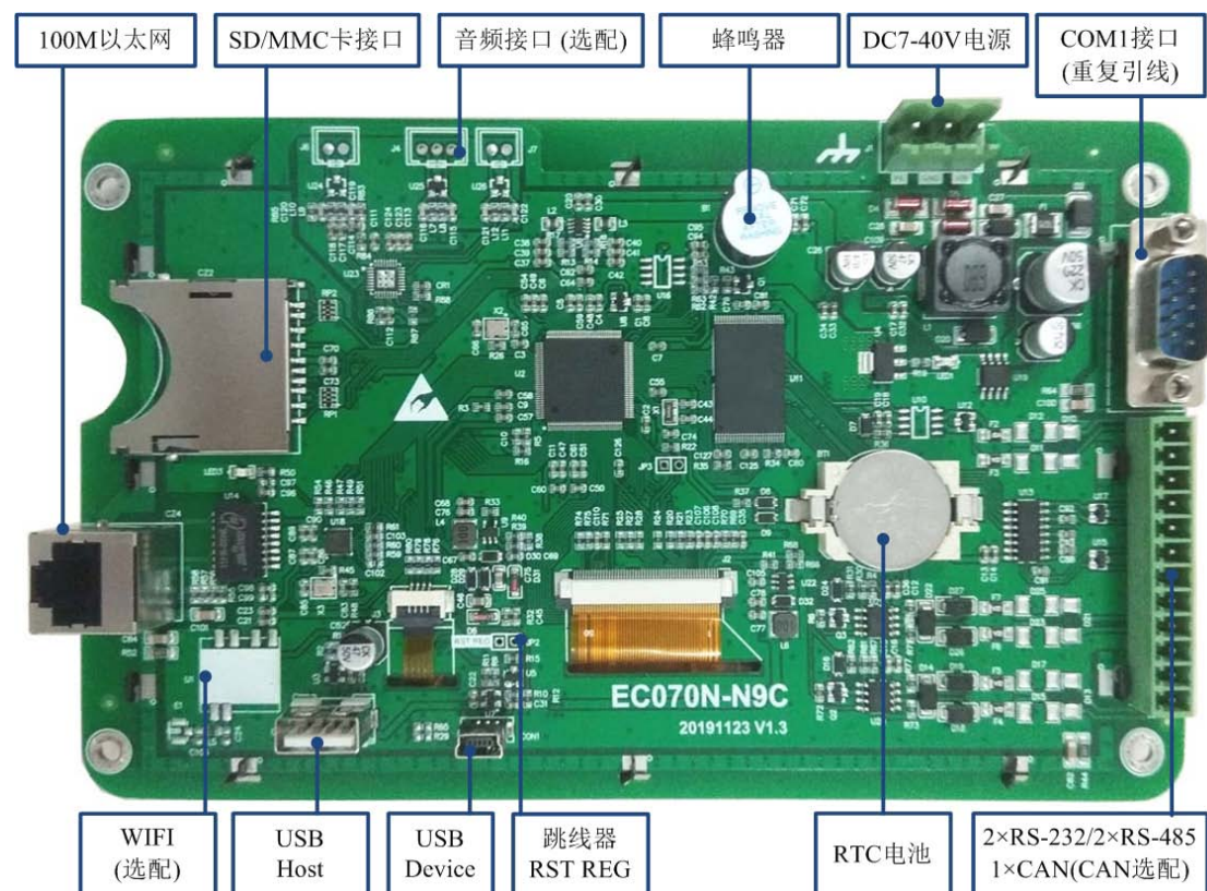
图 3.1 硬件接口概述
