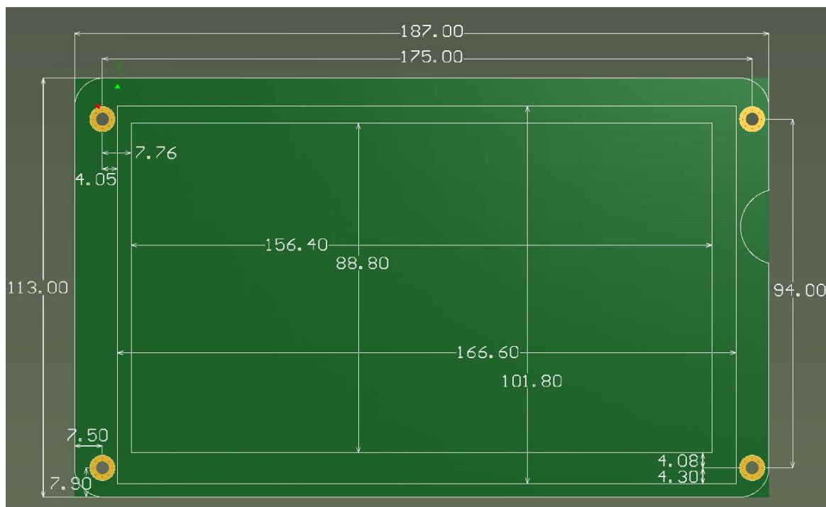
图 4.1 安装尺寸（单位 mm）
