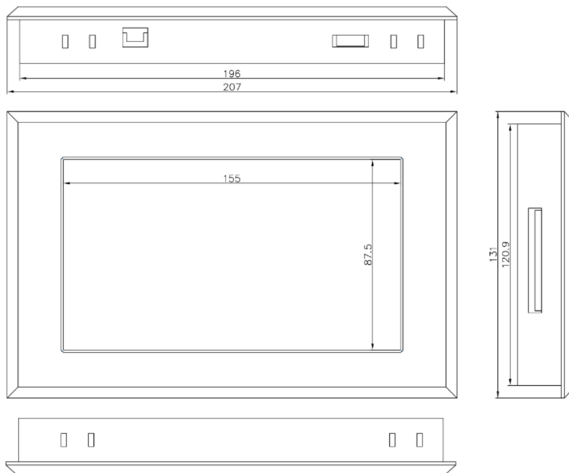
图 4.2 安装框尺寸（单位 mm）
